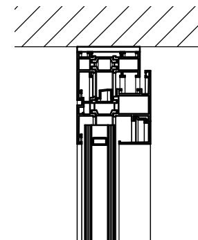
5 Detail 3 1 : 5
