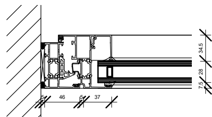
3 Detail 1 1 : 5
