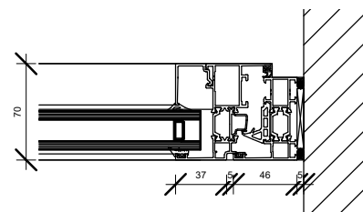
4 Detail 2 1 : 5
