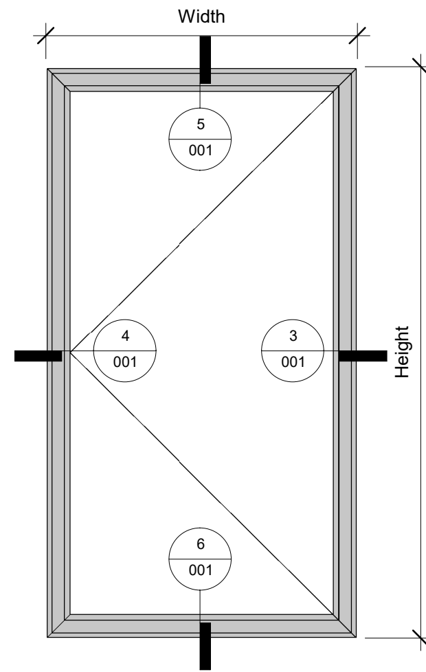
2 Elevation Back 1 : 20
