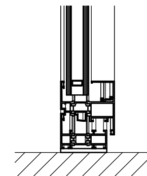
6 Detail 4 1 : 5
